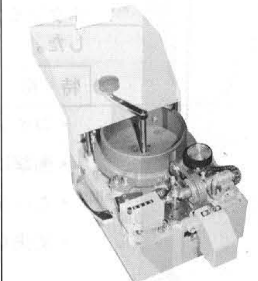
改良型(手動式) シュア-コインカウンター
