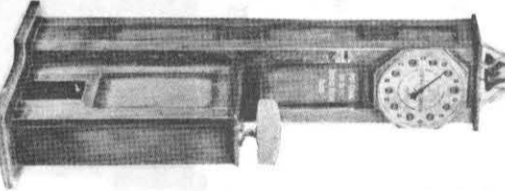
打力計 高さ二尺六寸 幅二尺 定価金四百八拾圓也
