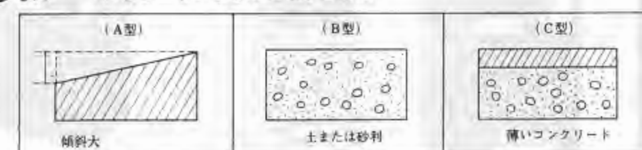
図：参考例 コンクリート工事を必要とするもの
